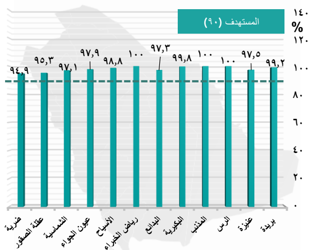
نسبة توصيل الإنترنت للمنازل بجميع وسائل الاتصالات
